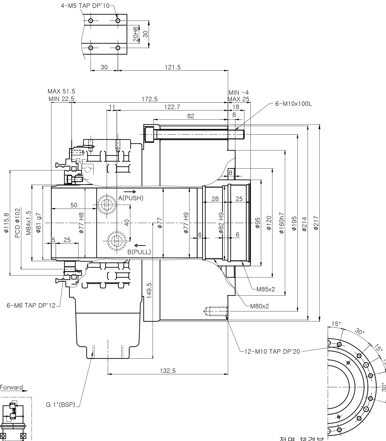
전면 체결부
