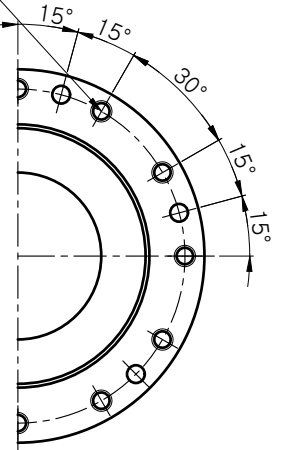
전면 체결부
